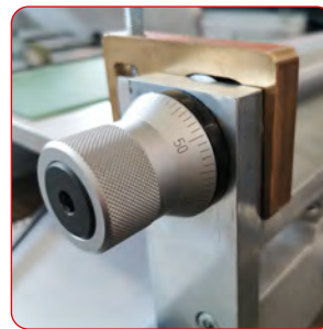
Regulación del ángulo de biselado.
