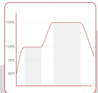
Zwei Temperaturhaltestufen.
